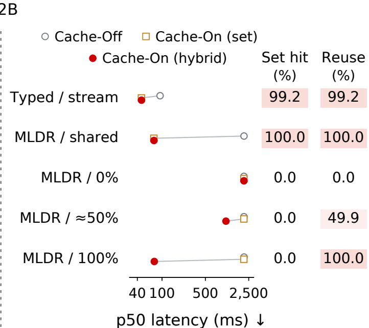
(d) Cacheable
