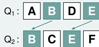
(d) Cacheable
